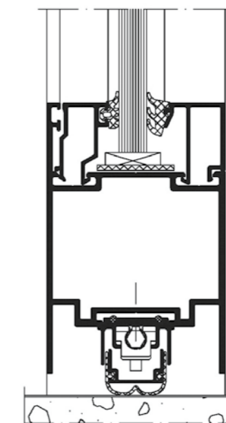
Porte Schüco ADS 65.NI FR 30
